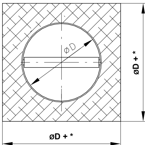
Maße der Einbauöffnung
