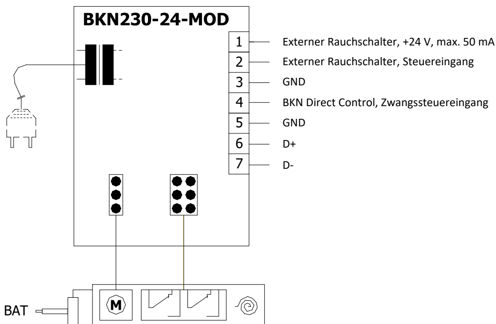
Kommunikations- und Stromversorgungseinrichtung BKN 230-24-MOD
