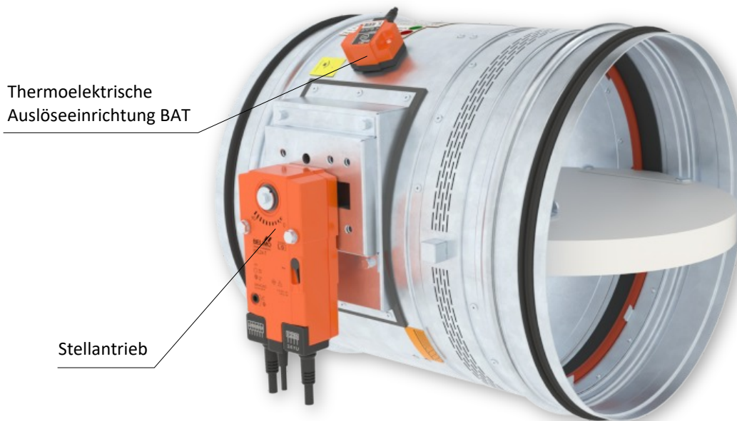
Ausführung .40 und .50
