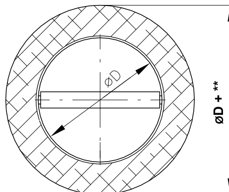
Maße der Einbauöffnung
