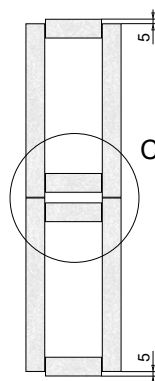
Aufbau der Distanzstreifen (H)
